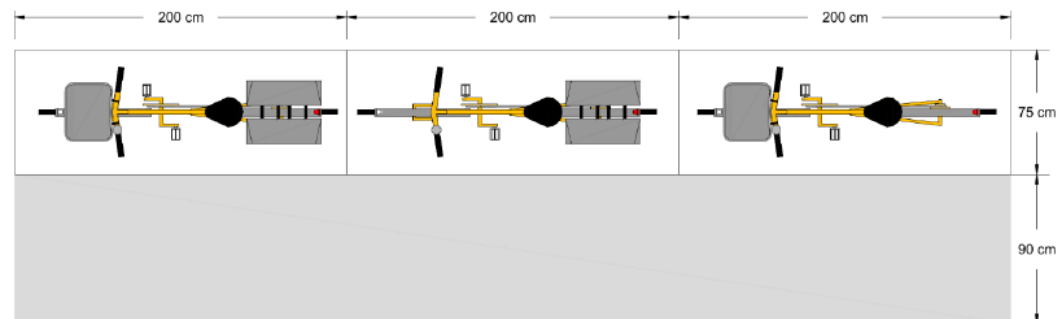
Figure 13 : Disposition longitudinale
